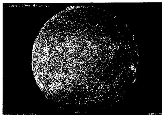
(Courtesy of National Solar Observatory and Kiepenheuer Institute für Sonnenphysik.)
