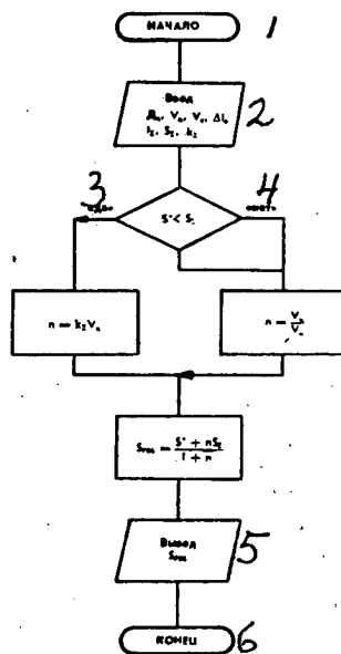
Рис. 1. Алгоритм программы.
