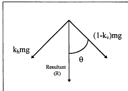
Fig 2-5b Mononobe-Okabe
