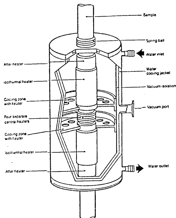
ZMF heater
