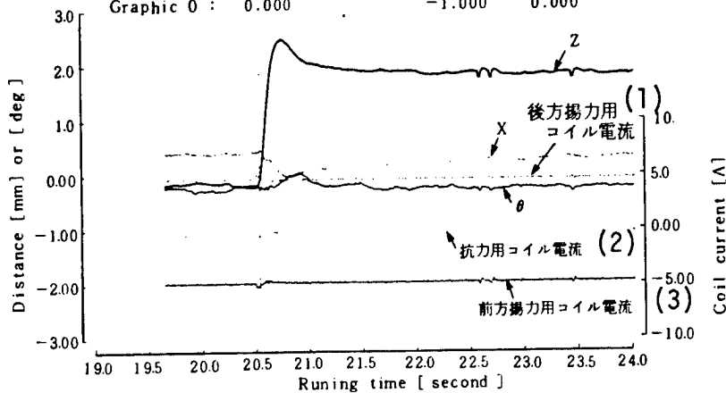
図4 磁力支持されている模型を2 mmだけ階段状に上昇させる命令を与えた時の模型の応答
