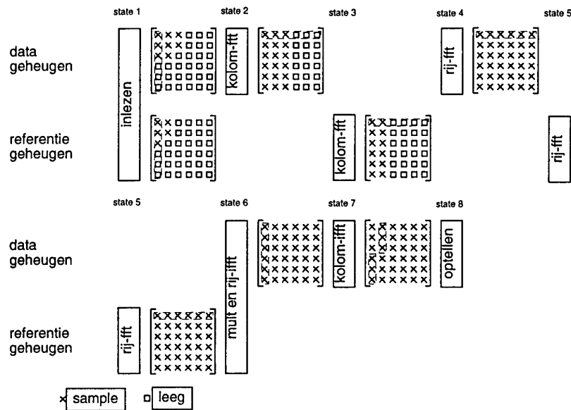
Figuur 3.10: Geheugenbehandeling per state. Data- en referentiegeheugen worden gepresenteerd als 6 \times 6 matrices. Ter illustratie is gekozen voor een data-reekslengte en referentiereekslengte van 8 respectievelijk 5 samples, en een 6 punts FFT. Dit impliceert dus een sectionering in secties bestaande uit 3 samples, 3 datasecties en 2 referentiesecties. Elke matrix in de figuur representeert het respectievelijke data- of referentiegeheugen 'nadat' de bewerking gedurende een state heeft plaatsgevonden. Bovendien wordt d.m.v. balken in de matrices aangegeven op welke 'wijze' (d.w.z. koloms- of rijgewijs of als half versprongen kolommen) de geheugenelementen beschikbaar zijn voor de volgende bewerking. De lege geheugenplaatsen worden bij het uitlezen vervangen door nullen (zero-padding).
