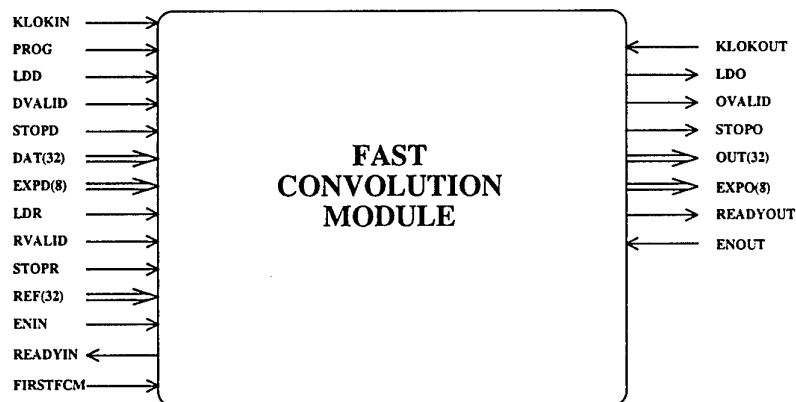
Figuur 2.6: Input/output signalen van de FCM.
