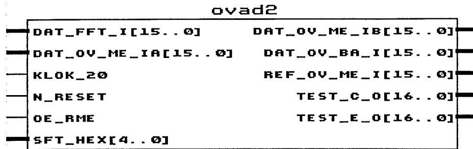
Figuur C.6: FPGA die zorgt voor het optellen van twee imaginaire reeksen tijdens kolom IFFT.
