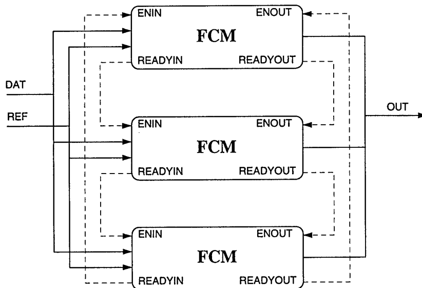
Figuur 2.4: Parallel schakelen van FCMs.
