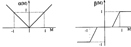
FIG. 5. Diffusion Coefficients.
