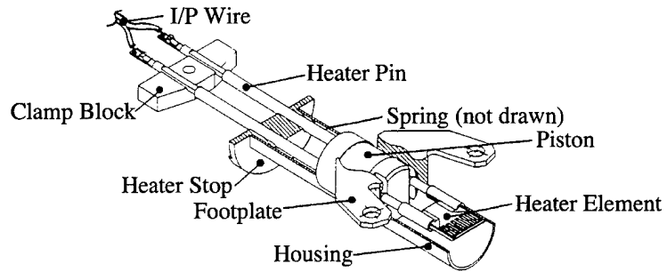
a. Fokker thermal knife.
