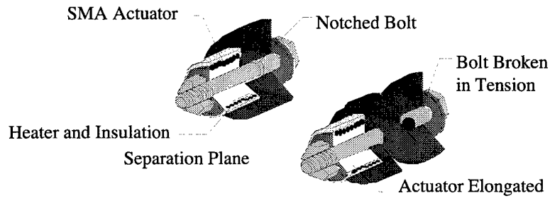
b. Ti-Ni Frangibolt.
