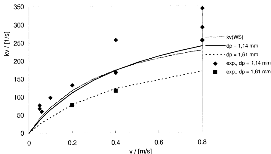
Figuur 3: Overall adsorptiesnelheidscoëfficiënt versus de superficiële gassnelheid. Experimenteel bepaalde waarden, \blacklozenge : d_p = 1,14 en \blacksquare : d_p = 1,61 mm, vergeleken met berekeningen volgens het model van Wood en Stampfer (vergelijking 5, grijze lijn) en volgens het in dit rapport gepresenteerde model (vergelijking 6), getrokken lijn voor d_p = 1,14 en stippellijn voor 1,61 mm.
