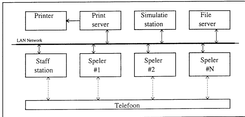
Figuur 3.4: Fysieke layout van AOW-II.
