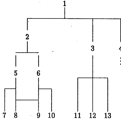
Fig. 2.2. DAG for Example 2.0.1.
