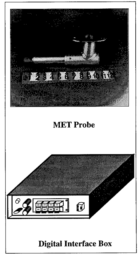
Figure 5-2 MET Sensor
