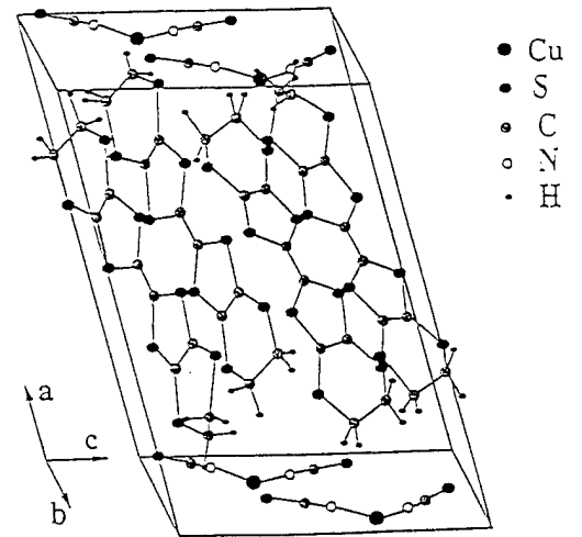
ET 2 Cu(NCS) 2 Structure
