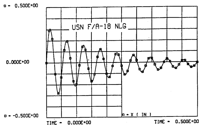
Fig. 9a. Simulation of F/A-18A (USN)
