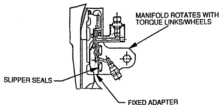
Fig. 7. Steering Manifold
