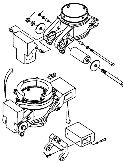
Fig. 8. Mass Damper
