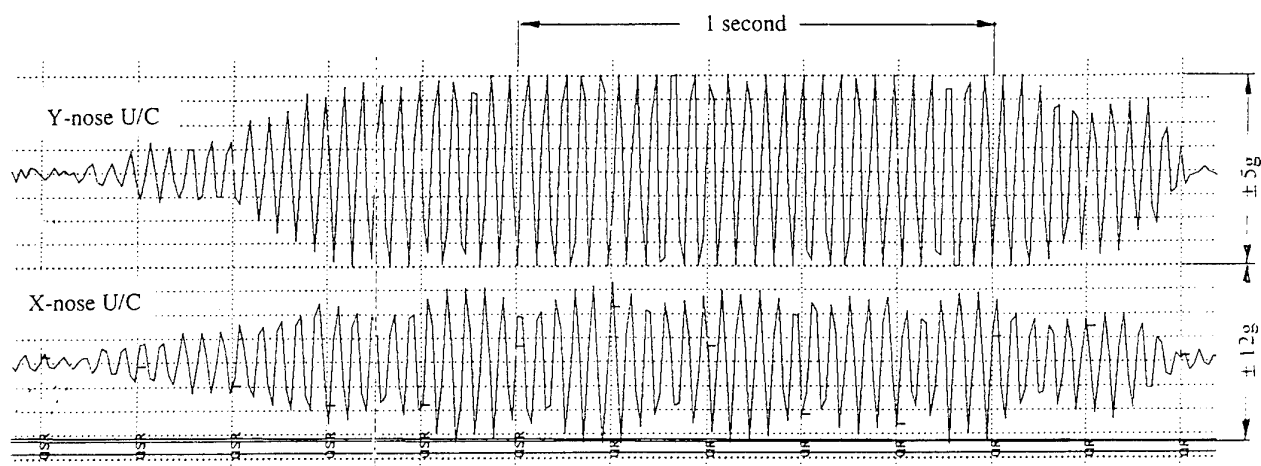
Fig. 2 - 4 Shimmy
