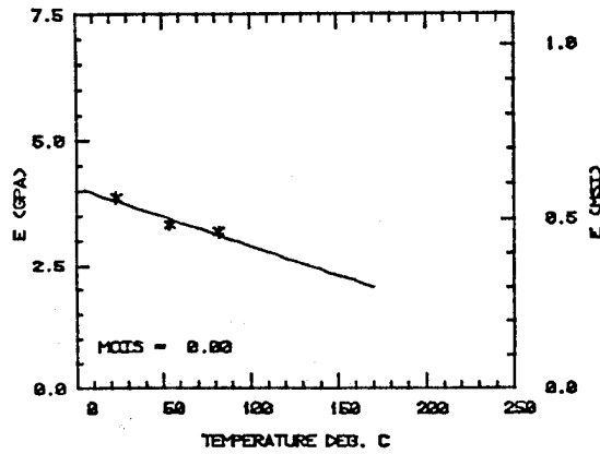
a) Hercules 3502
