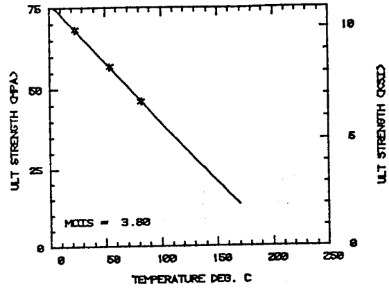
b) Hercules 2220-1
