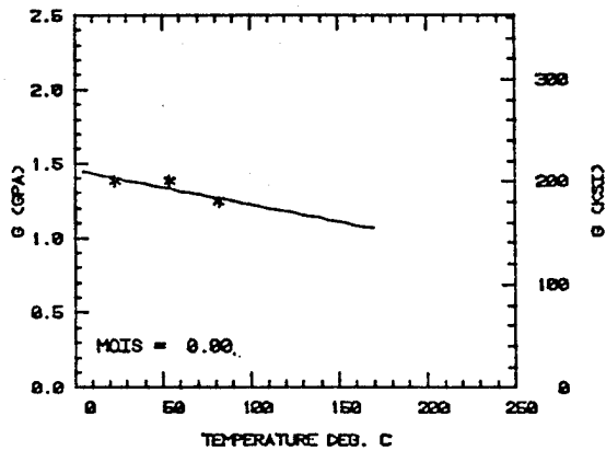
c) Hercules 2220-3
