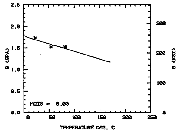
b) Hercules 2220-1
