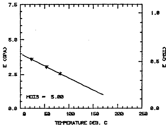
a) Hercules 3502
