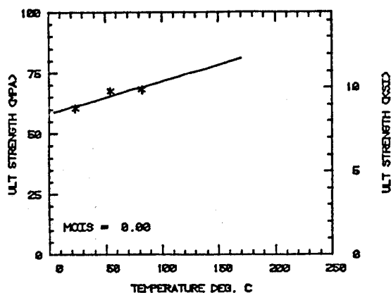
a) Hercules 3502
