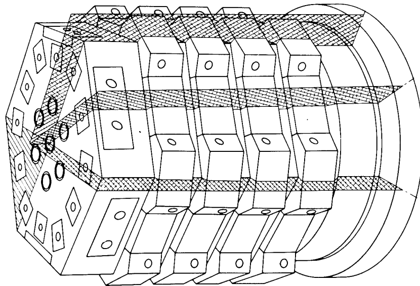
(a) Actual structure
