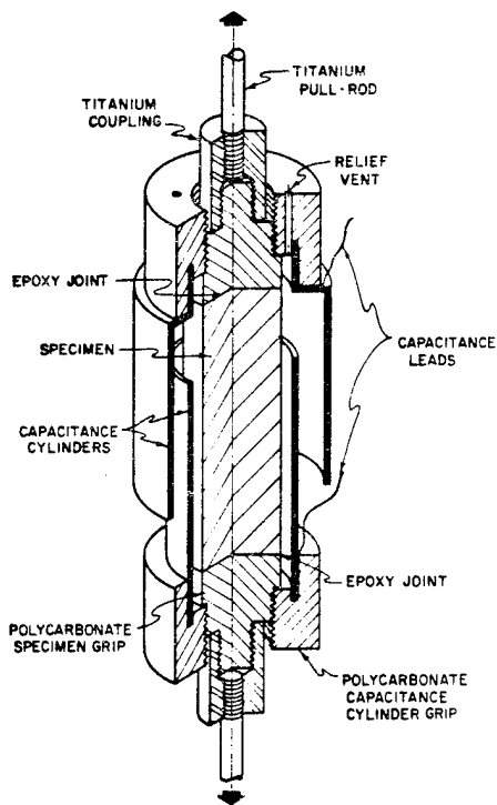
Tensile
