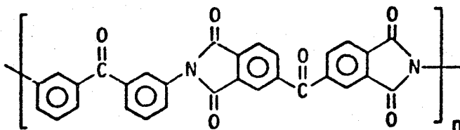
LARC-TPI
