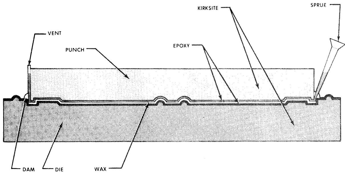
FIG.11 POUR EPOXY FACE ON PUNCH
