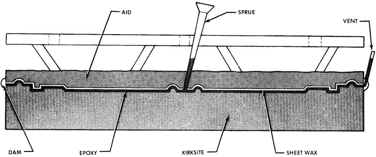
FIG. 10 POUR EPOXY FACE ON DIE
