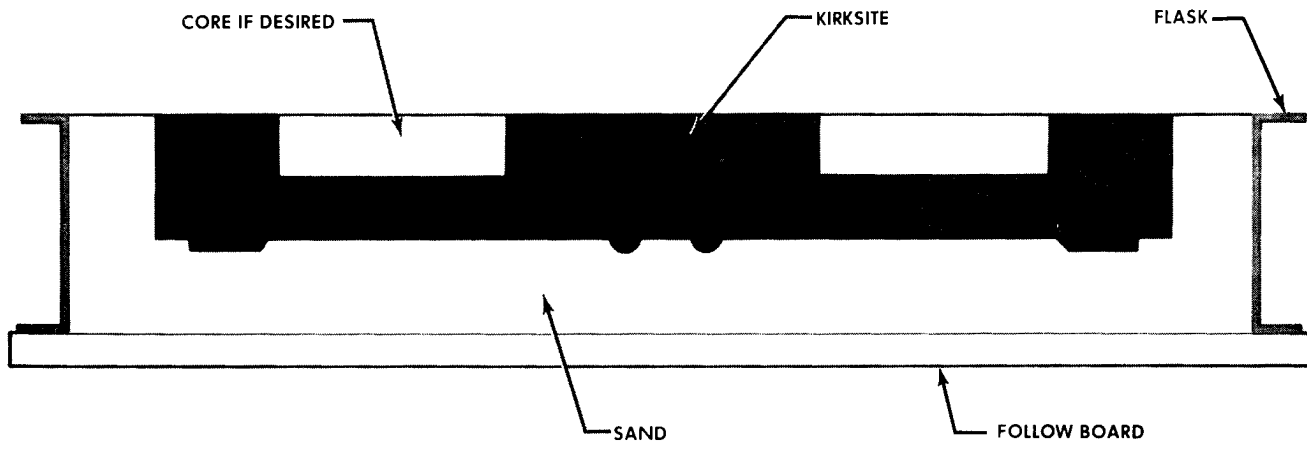
FIG. 3 POUR KIRKSITE IN OPEN SAND MOLD
