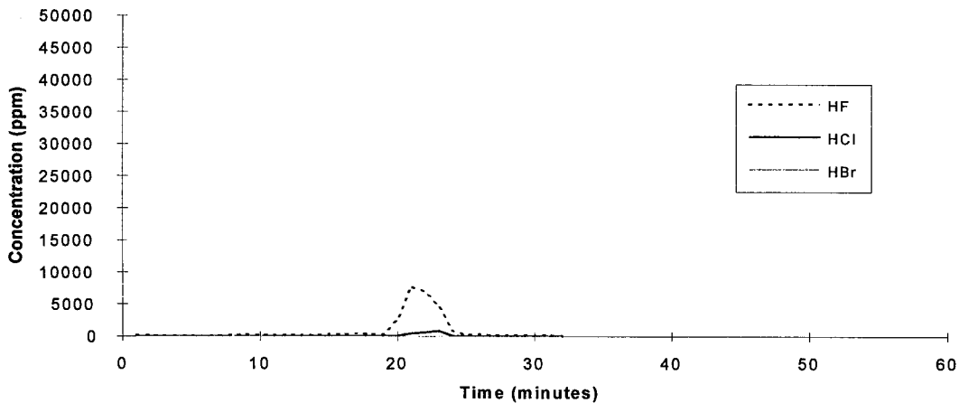
Halon 1301- Test 3
