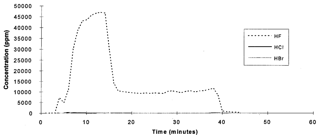
Perfluorohexane - Test 1
