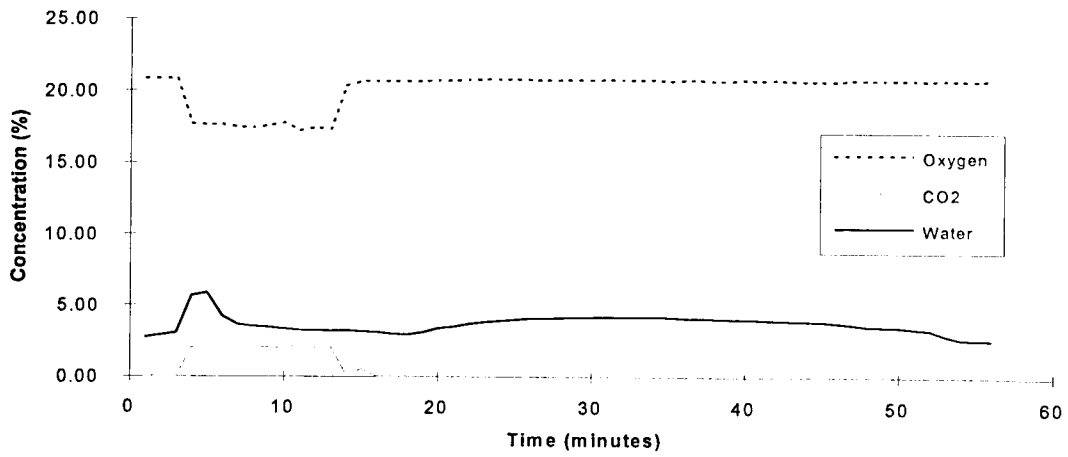
HFC -125 - Test 2
