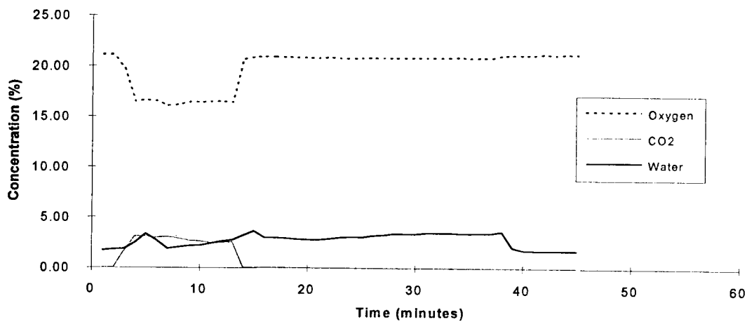
Perfluorohexane - Test 2
