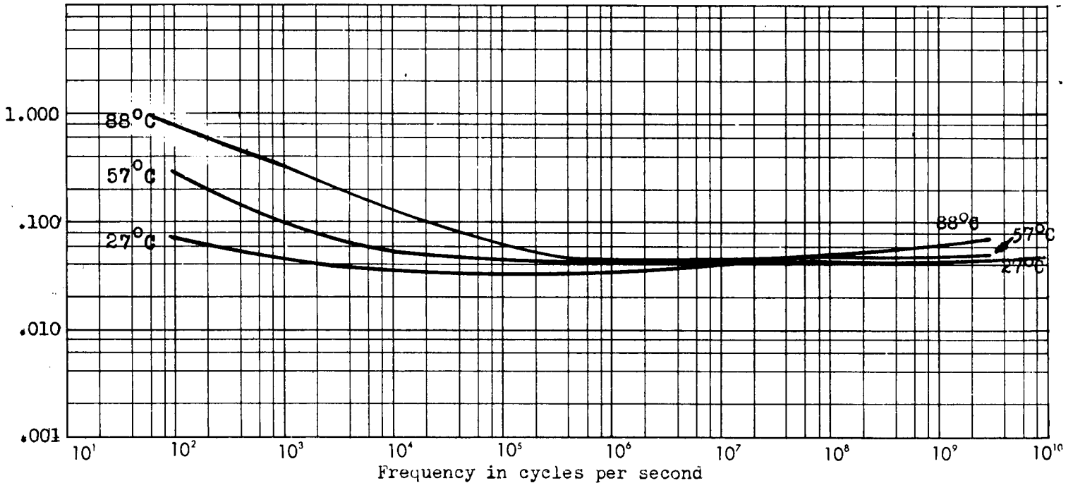
TAN δ
