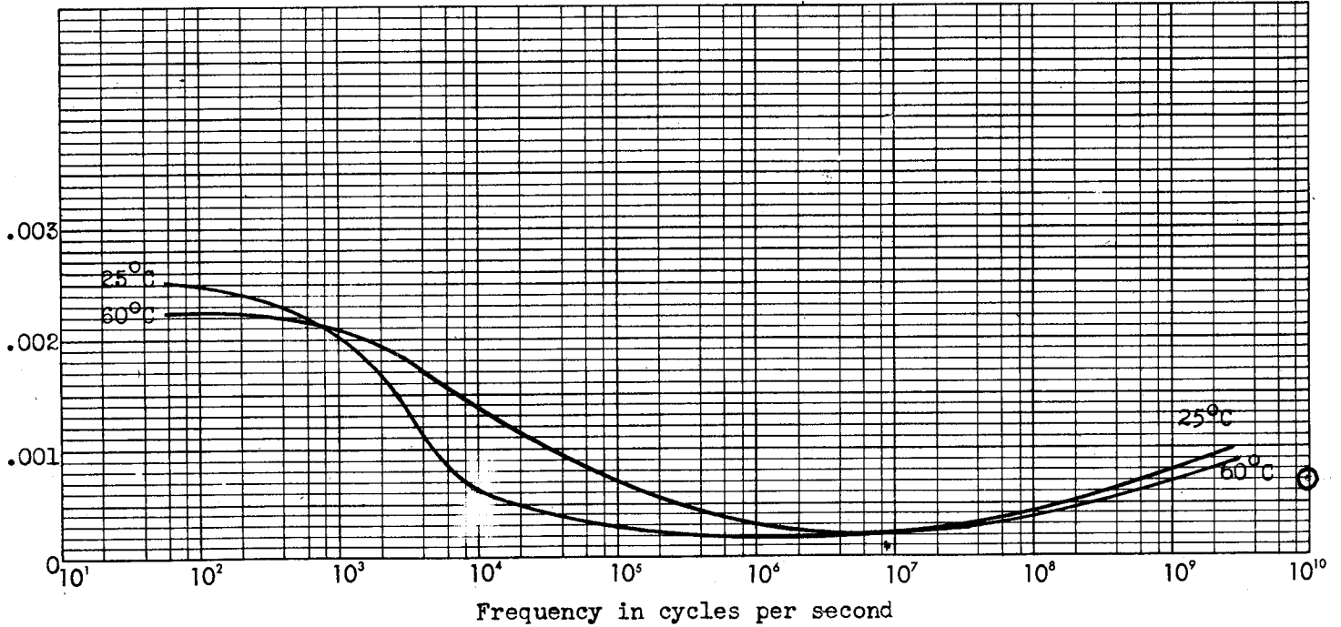
TAN \delta
