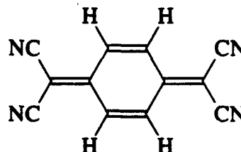
TCNQ
