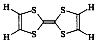
TTF
