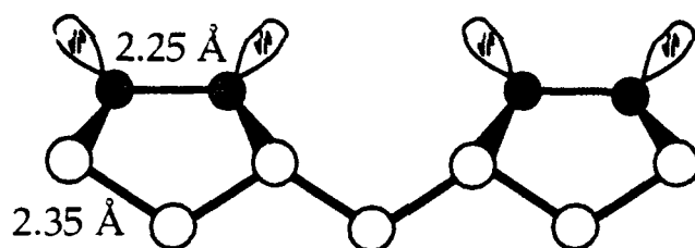
P-P dimer
