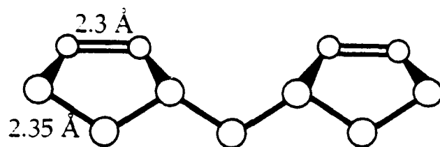
Si=Si dimer
