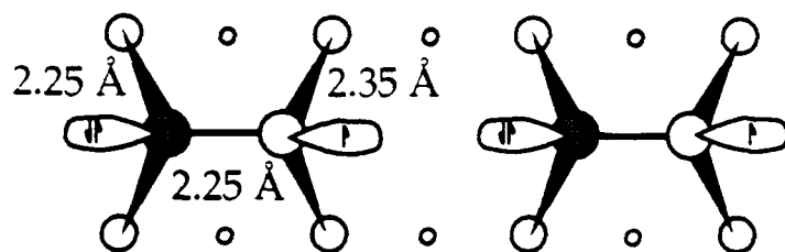
P-P dimer
