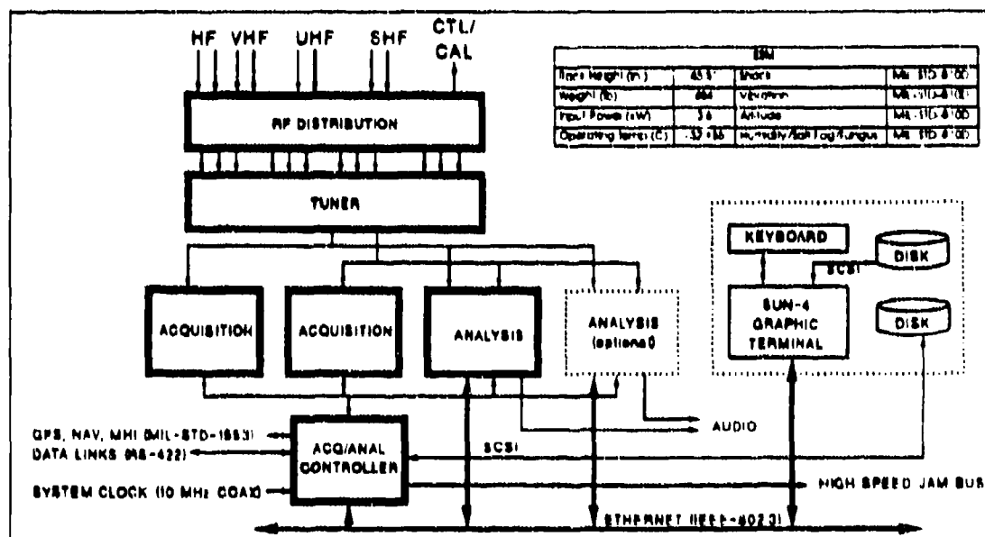
Figure 3-9. TACJAM-A Block Diagram
