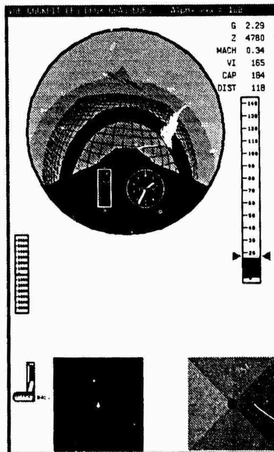
Figure 5 : Fenêtre vue Cockpit.
