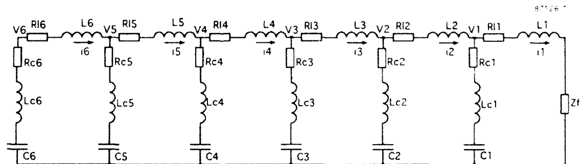
Figuur 7 Schema van het pulsvormende netwerk dat gebruikt wordt als energiebron voor de flitsbuis
