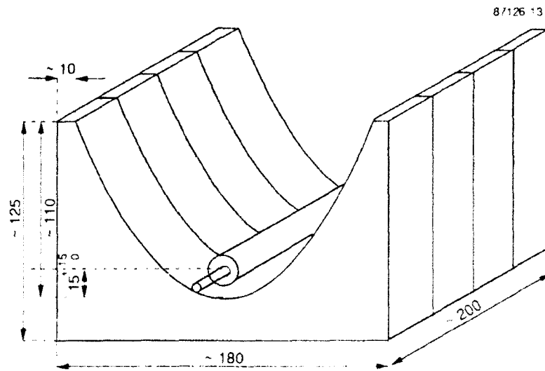
Figuur 13 Ontwerp van de parabolische reflector van de flitscr. Het spiegeloppervlak voldoet aan de vergelijking y = \frac{1}{60} x^2 (in mm). De brandpuntsafstand bedraagt derhalve 15 mm
