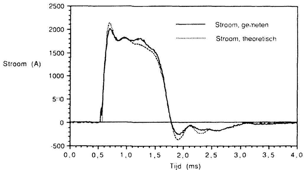
Figuur 24 Stroom door een flitsbuis met impedantie van 0,41 \Omega
