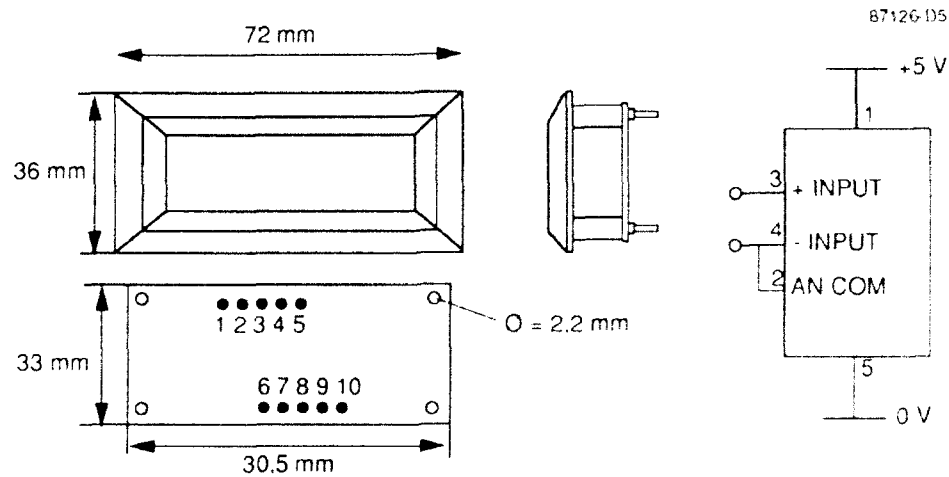
Figuur D5 Aansluitingen van de paneelmeeters
