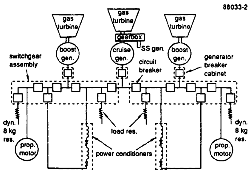
Figuur 2.4 Systeem met een gecombineerde elektrische voortstuwing
