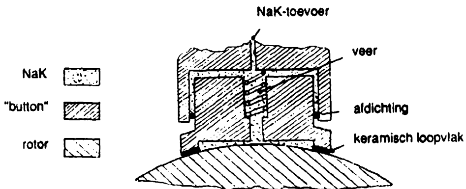
Figuur 4.9 NaK borstels van Garrett
