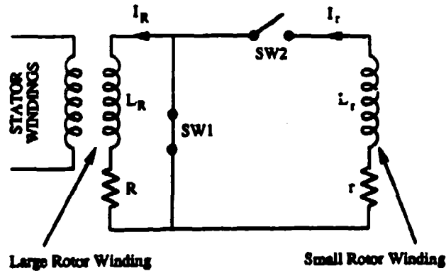
Figuur 4.2 Schematische voorstelling van de SEAC motor
