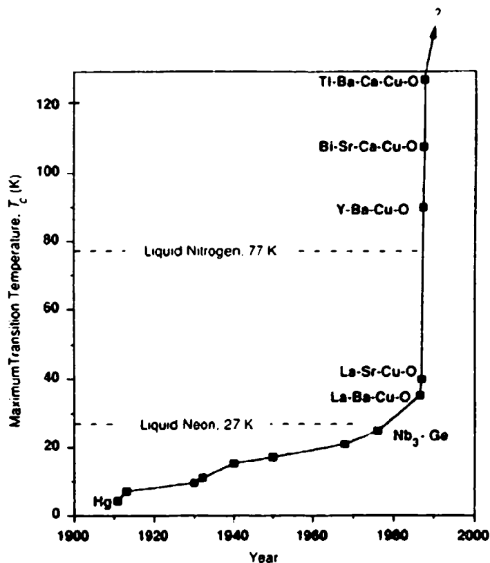
Figuur 3.4 Ontwikkeling van de hoge-temperatuur supergeleiders
