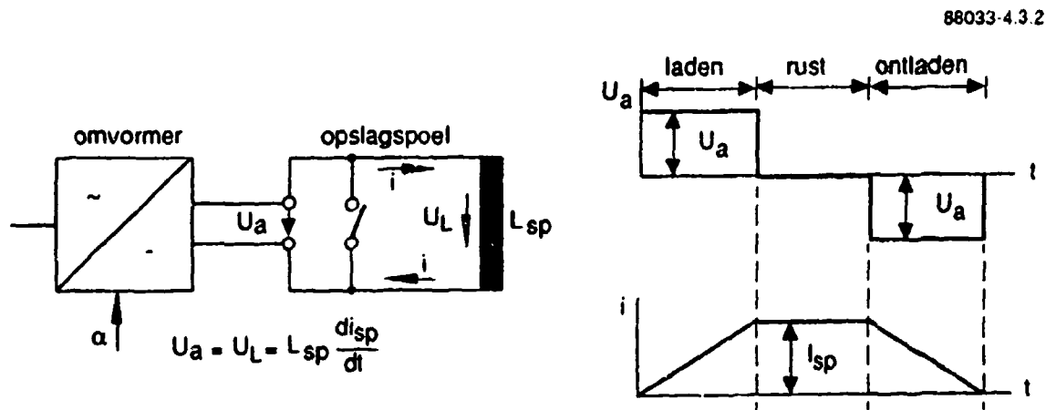
Figuur 4.3.2 Het laden en ontladen van een opslagspoel door een direkte aansluiting van een spanningsbron
