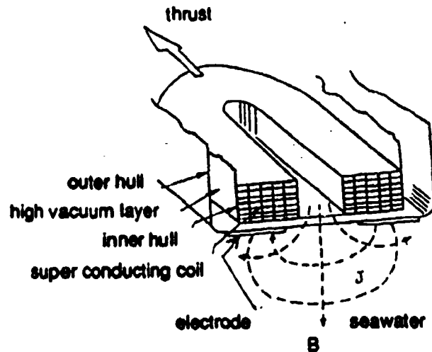
Figuur 4.15 EM-voortstuwning met een DC magnetisch veld waarbij de elektroden zich aan de buitenkant van het schip bevinden
