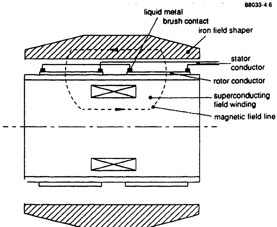
Figuur 4.6 Homopolaire generator met een drumrotor
