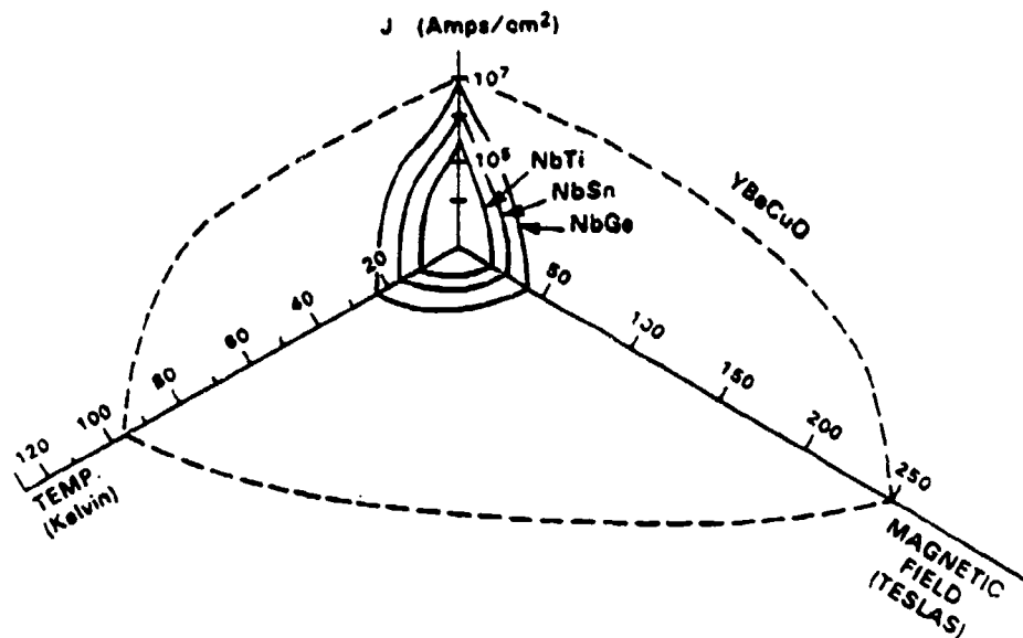
Figuur 3.1 De kritische waarden voor J, H, T
