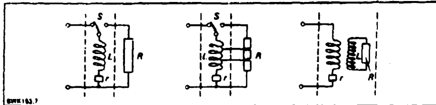
Figuur 4.3.4 Beveiliging van een supergeleidende spoel
