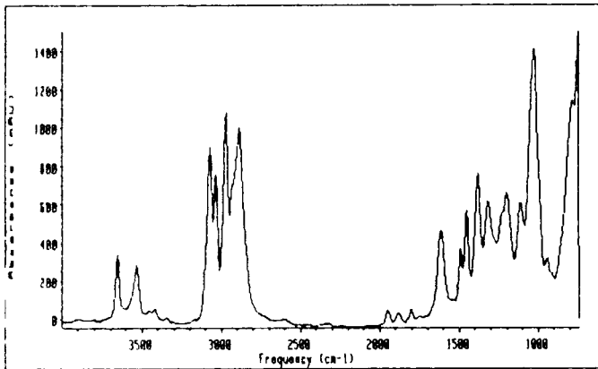
Phenylpropanolamine
