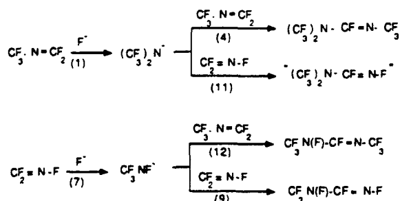
Scheme VI
