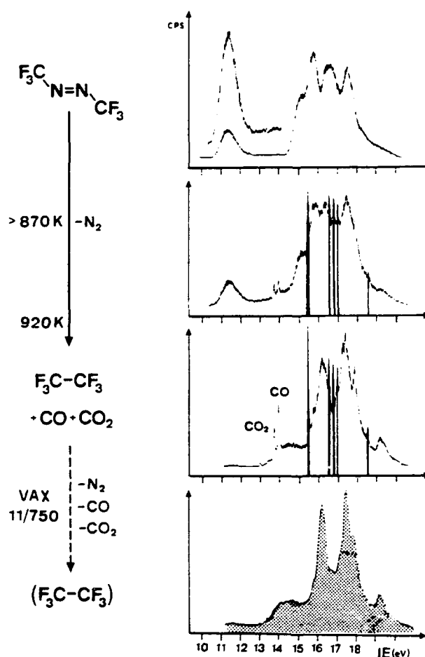
Abb. 3. He(I)-PE-Spektren von trans -Hexafluorazomethan und der bei Pyrolyse im externen Quarzrohr bei 880 K und 920 K entstehenden Produkte (vgl. Text, N_2 -Banden schwarz). Computer-Subtraktion der Ionisationsmuster von N_2 , CO und CO_2 liefert das schraffierte Spektrum, welches nach Literaturvergleich [23] Hexafluorethan zuzuordnen ist.
