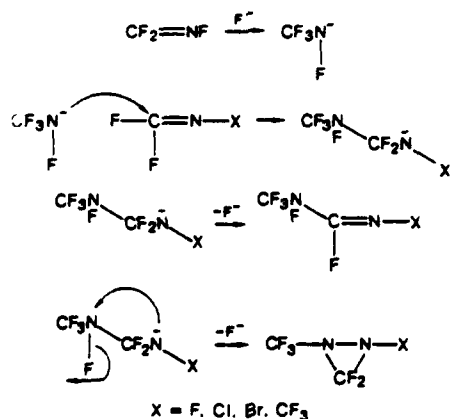
Scheme VI
