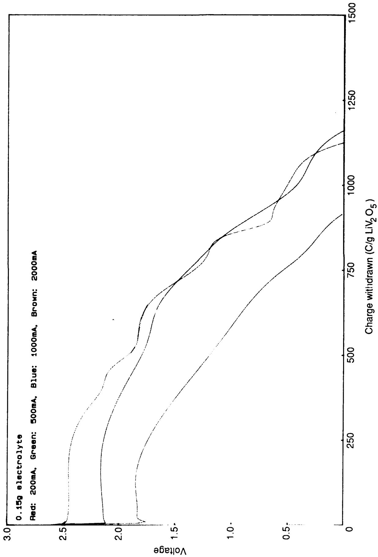
Fig 12 \text{LiV}_2\text{O}_5 500C
