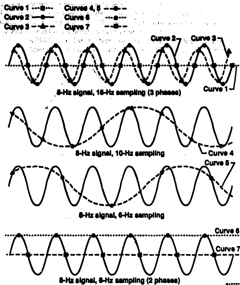
Figure 3-8. Sampling data.
