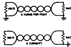
Fig. 2.5.1 Twisted pair
