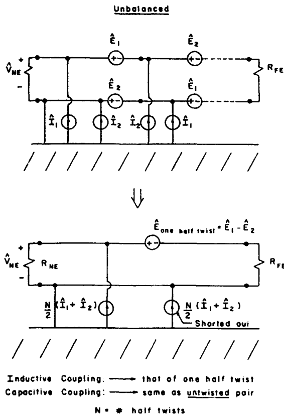
Fig. 21. Untwisting the twisted pair
