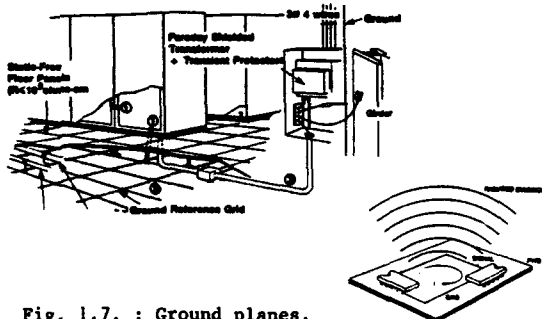
Fig. 1.7. : Ground planes.
