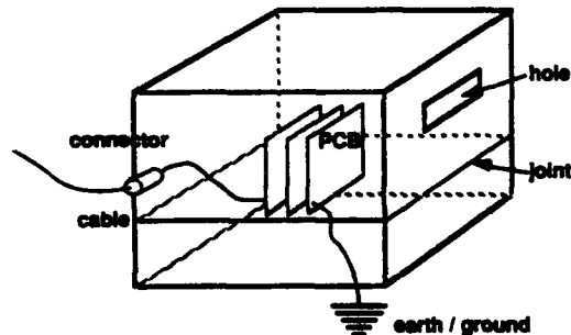
Fig. 2.3.1. : Real shielded boxes.
