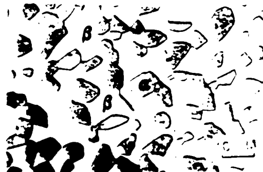
Alloy 4 ( 45 % \alpha + 55 % \beta )
