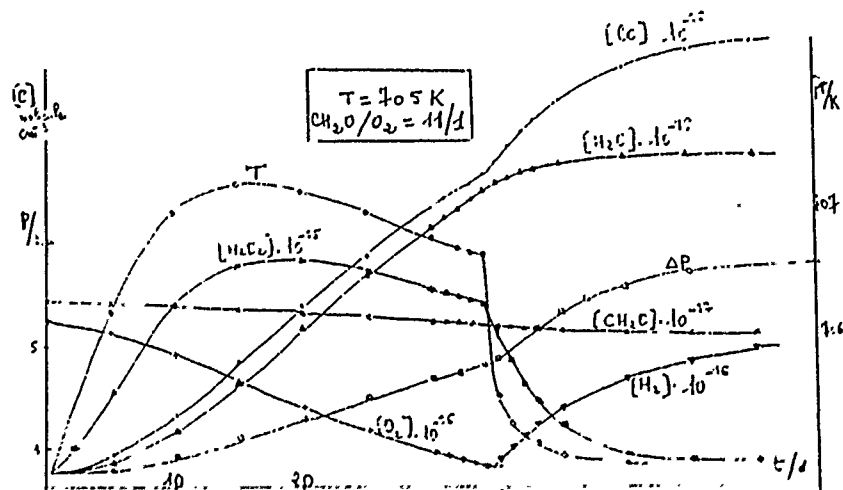
Fig 3 - Combustion calculées
