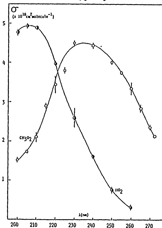
FIG. 1 : U.V. SPECTRA OF CH 3 O 2 AND HO 2 .
