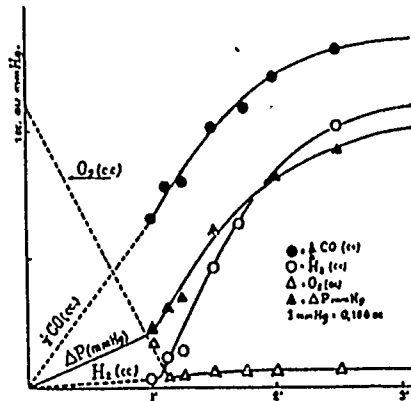
Fig. 1 — Analyse des produits de la réaction du mélange 8,7 mm O_2 + 66,3 mm CH_2O à 870^\circ C . Chambre de réaction pyrex : \phi : 4,8 cm, longueur : 20 cm. Les quantités de gaz sont exprimées en cc ramené à 0^\circ C et 760 mm Hg. La pression est exprimée en mm Hg à la température de 870^\circ C .
