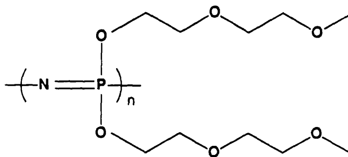
Poly[bis(2-(2-methoxyethoxy)ethoxy)phosphazene]
