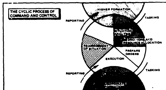
Fig. 2 C2-cyclus
