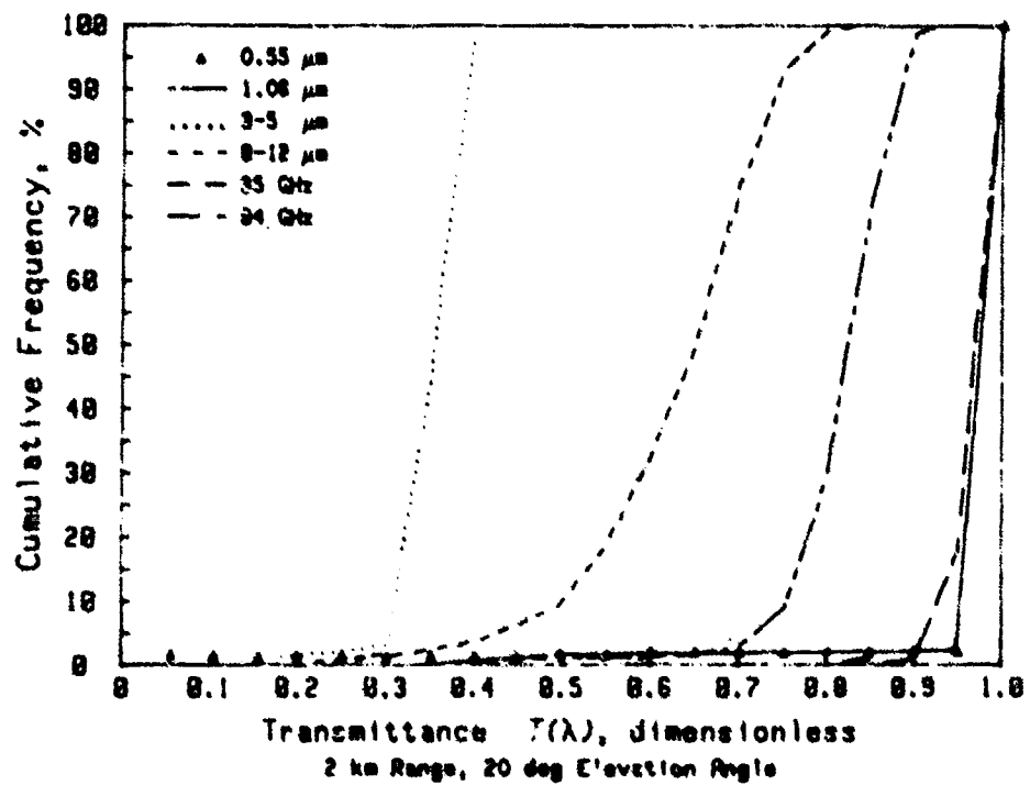
(D) Efsahan, Iran, 2400 Hours
