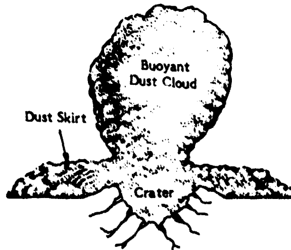
(B) Rise Phase
