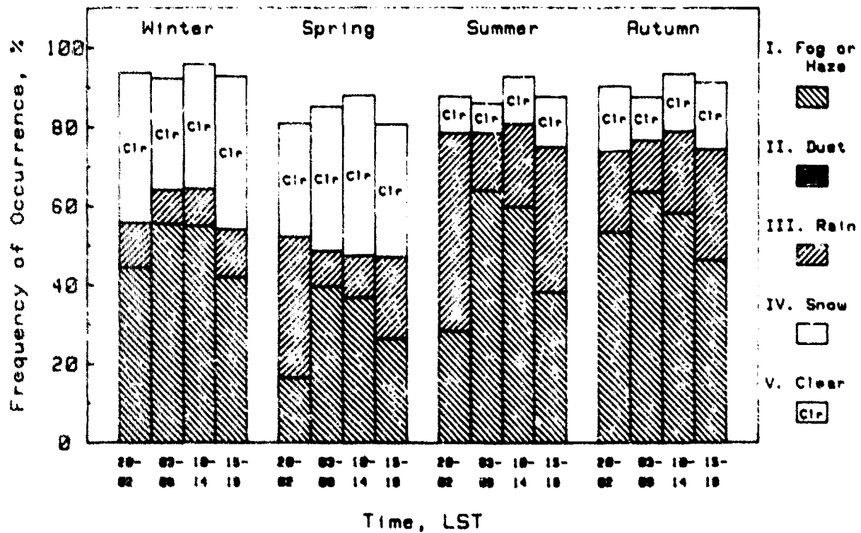
(D) Visibility 7 km or Greater
