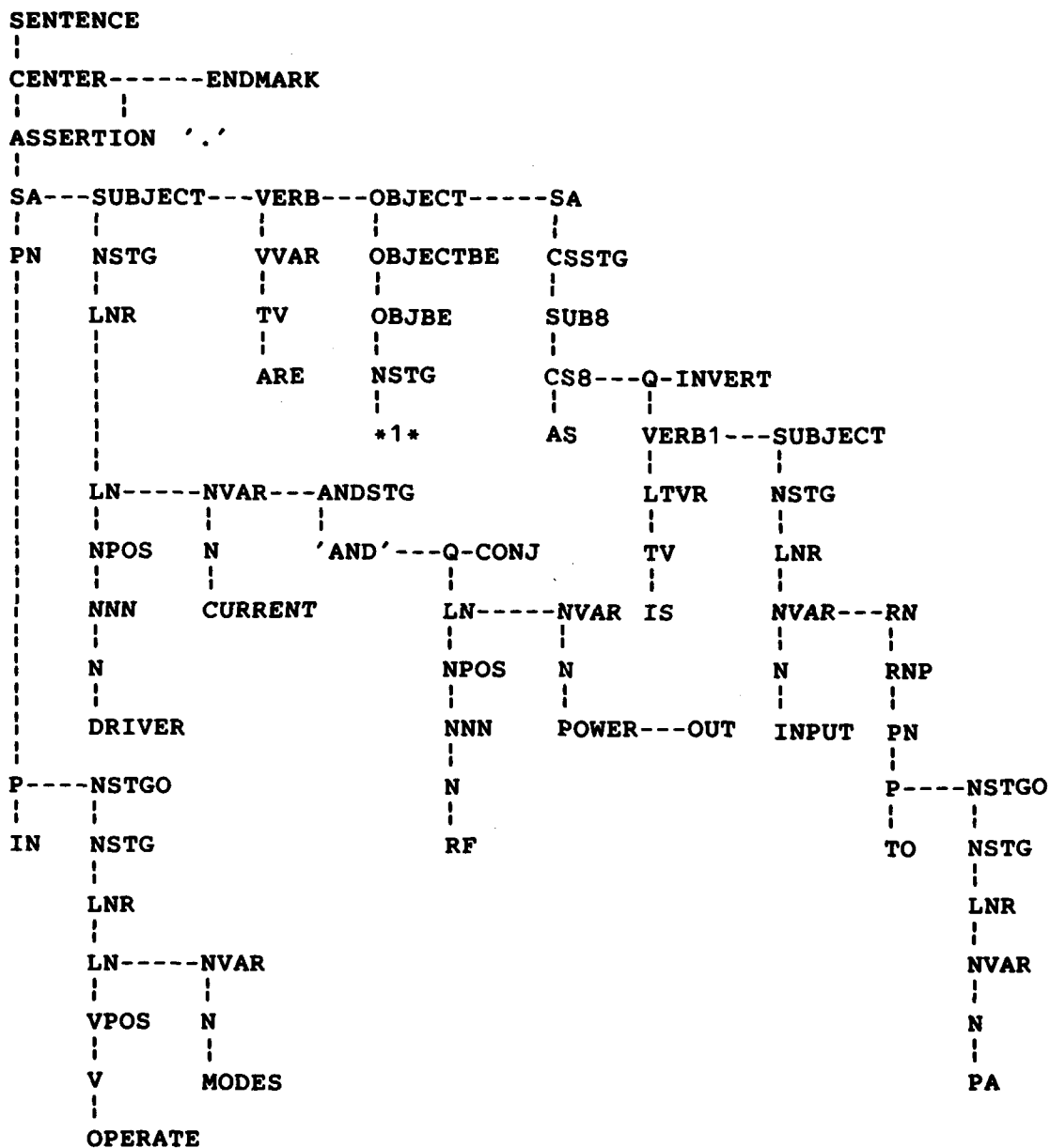
Fig. 2 - Parse tree
