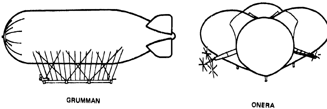
Fig. 3.12 Multielement concepts
