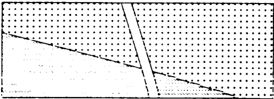
3. Intrude Mafic-Igneous
