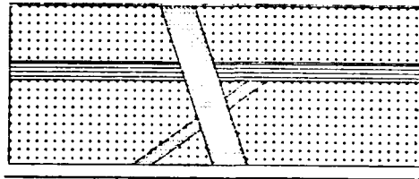
7. Erode
