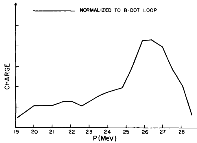
Fig. 9. Charge-vs-momentum.
