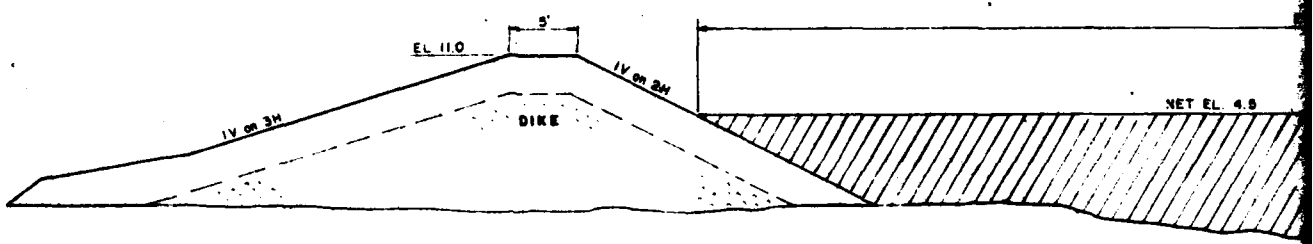
SECTION A-A
