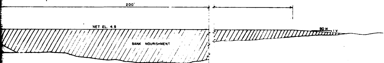
SECTION A-A
