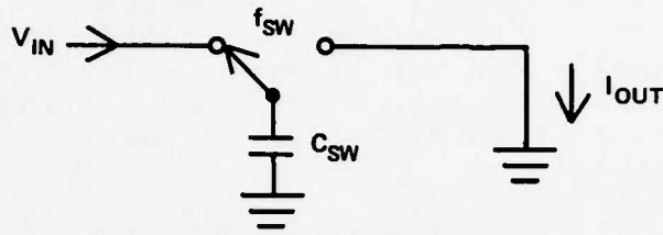
A. CIRCUIT
