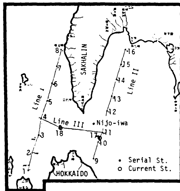
第 1 圖 宗谷海峽調査地點及航路圖
