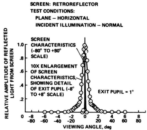
Fig. 51 Test data, retro-reflective screen
