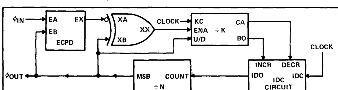
(d) ECPD WITH RIPPLE CANCELLATION
