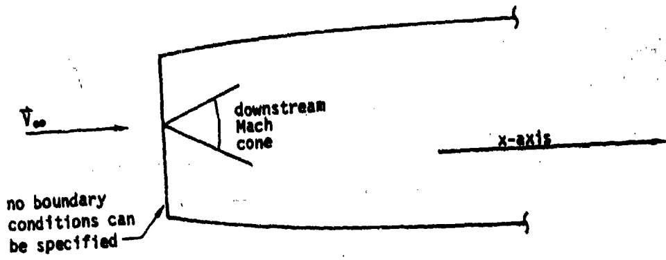
a) nacelle inlet
