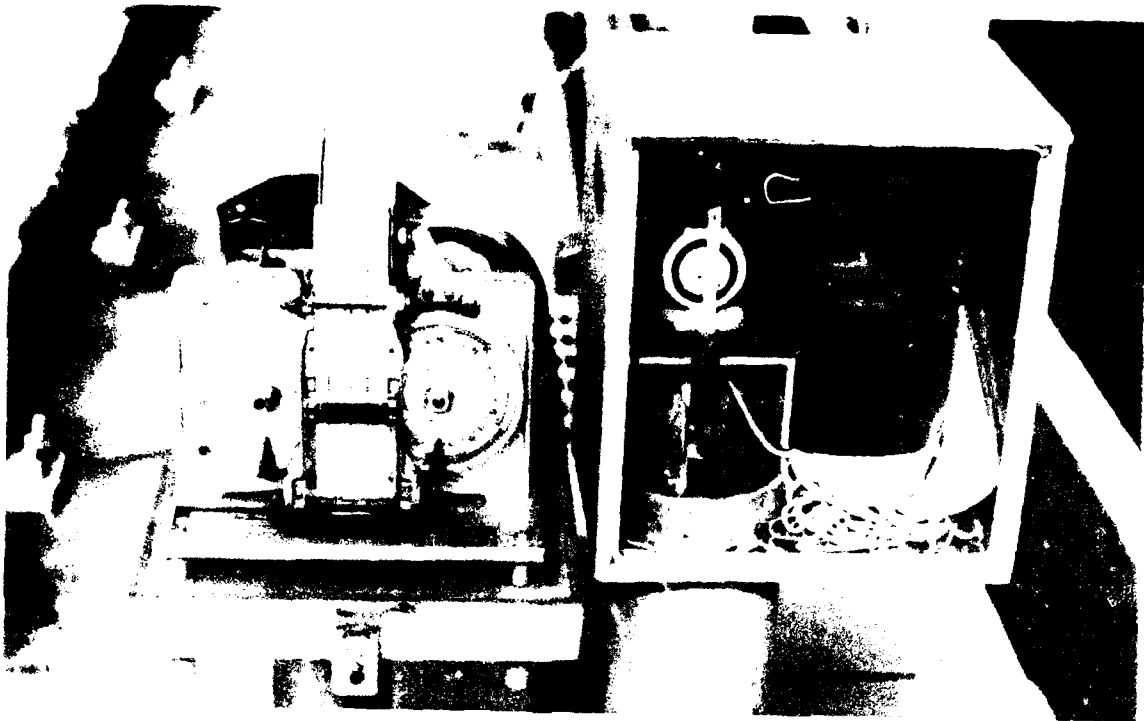
Figure 16. Fischer-Porter tide gage.
