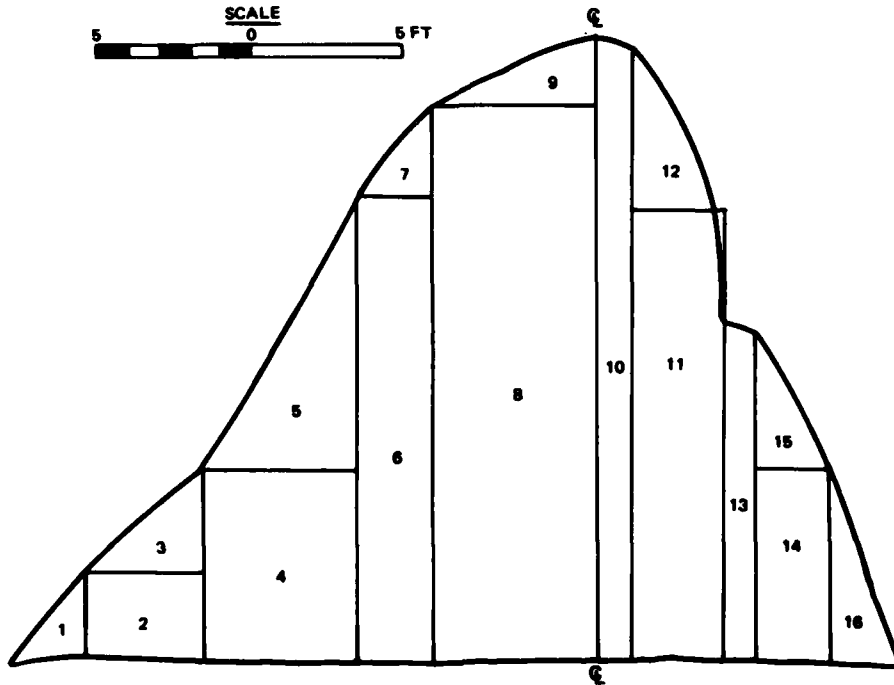
b. SECTION A2 - A4
