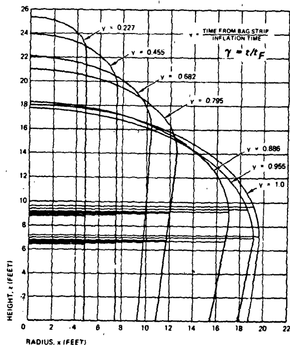
a) Canopy Profiles
