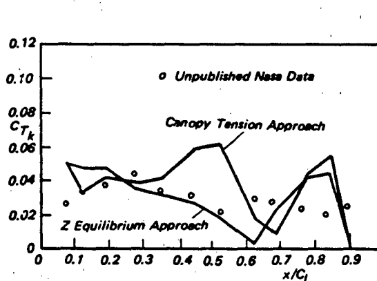
a) Keel Line Loads
